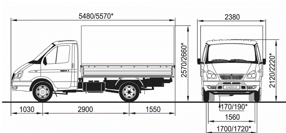
Рисунок 6.1 - Автомобіль ГАЗ – 3302
