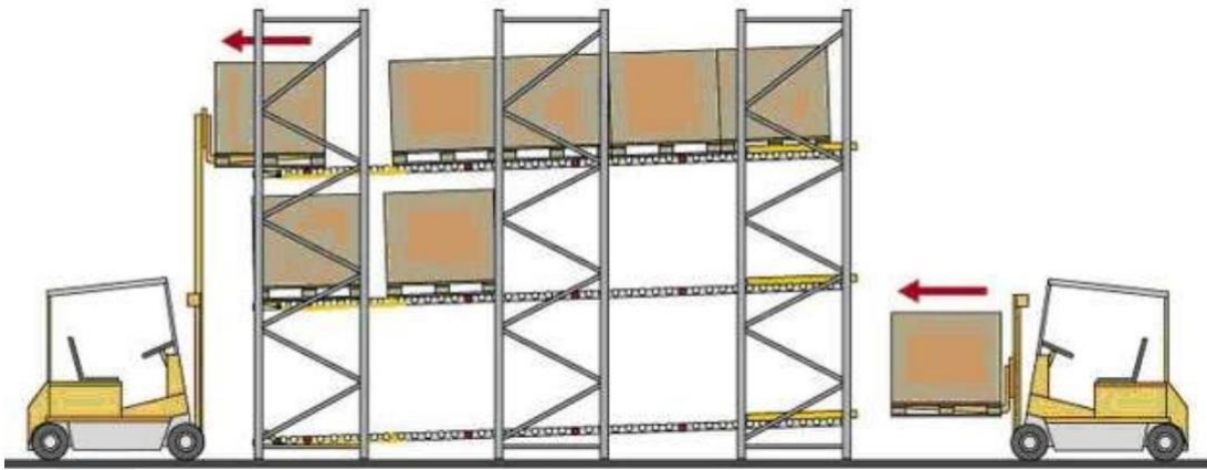
Рисунок 2.2 – Принцип роботи гравітаційного стелажа (приклад).
