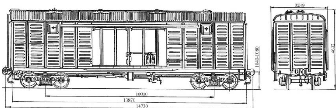
Рисунок 2.6-Чотирирівнісний критий суцільно-металевий вагон з розширеними дверними отворами модель 11 217 13 (приклад)
